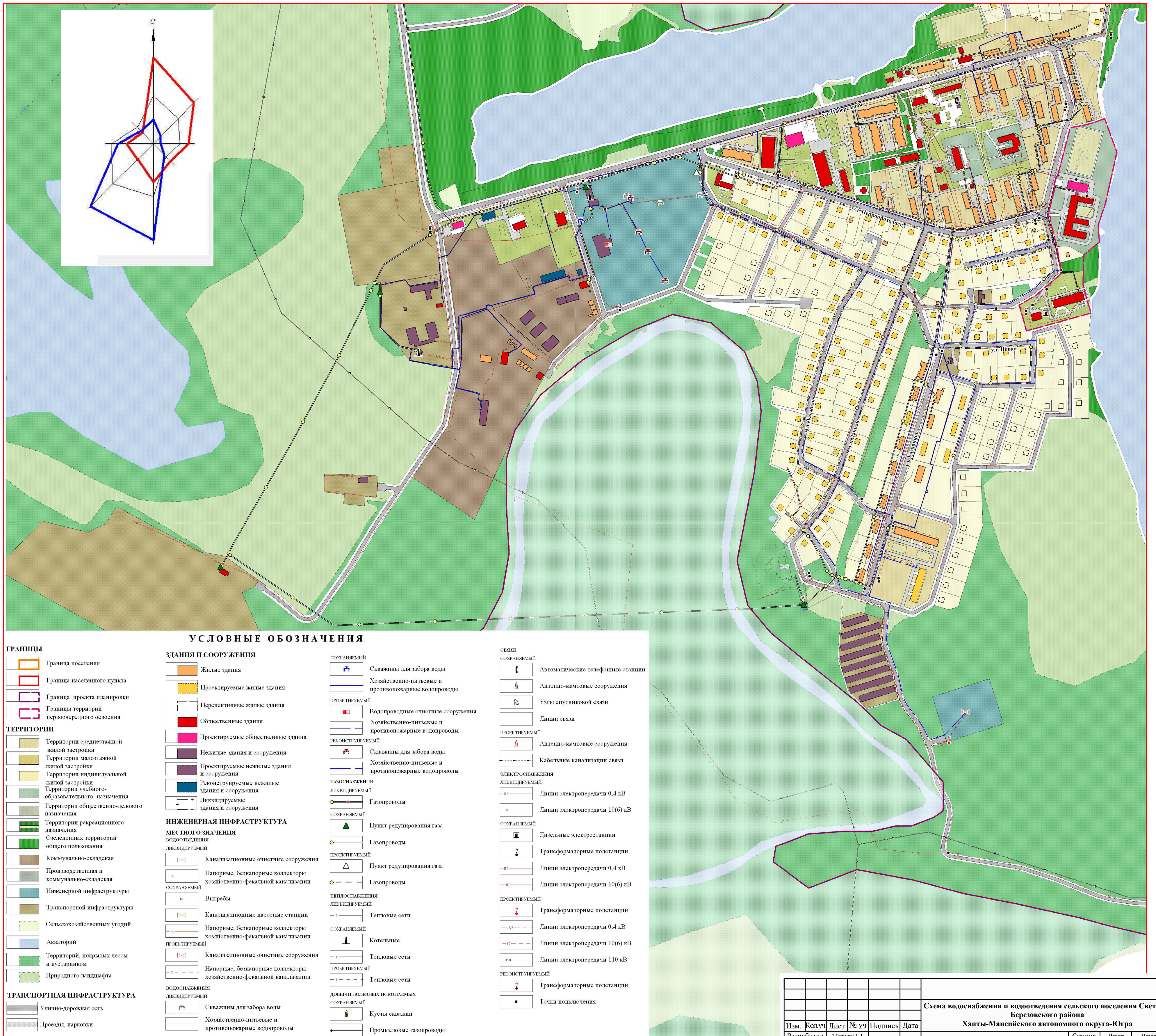
Схема водоснабжения и водоотведения п. Светлый фрагмент территории М1:5000
